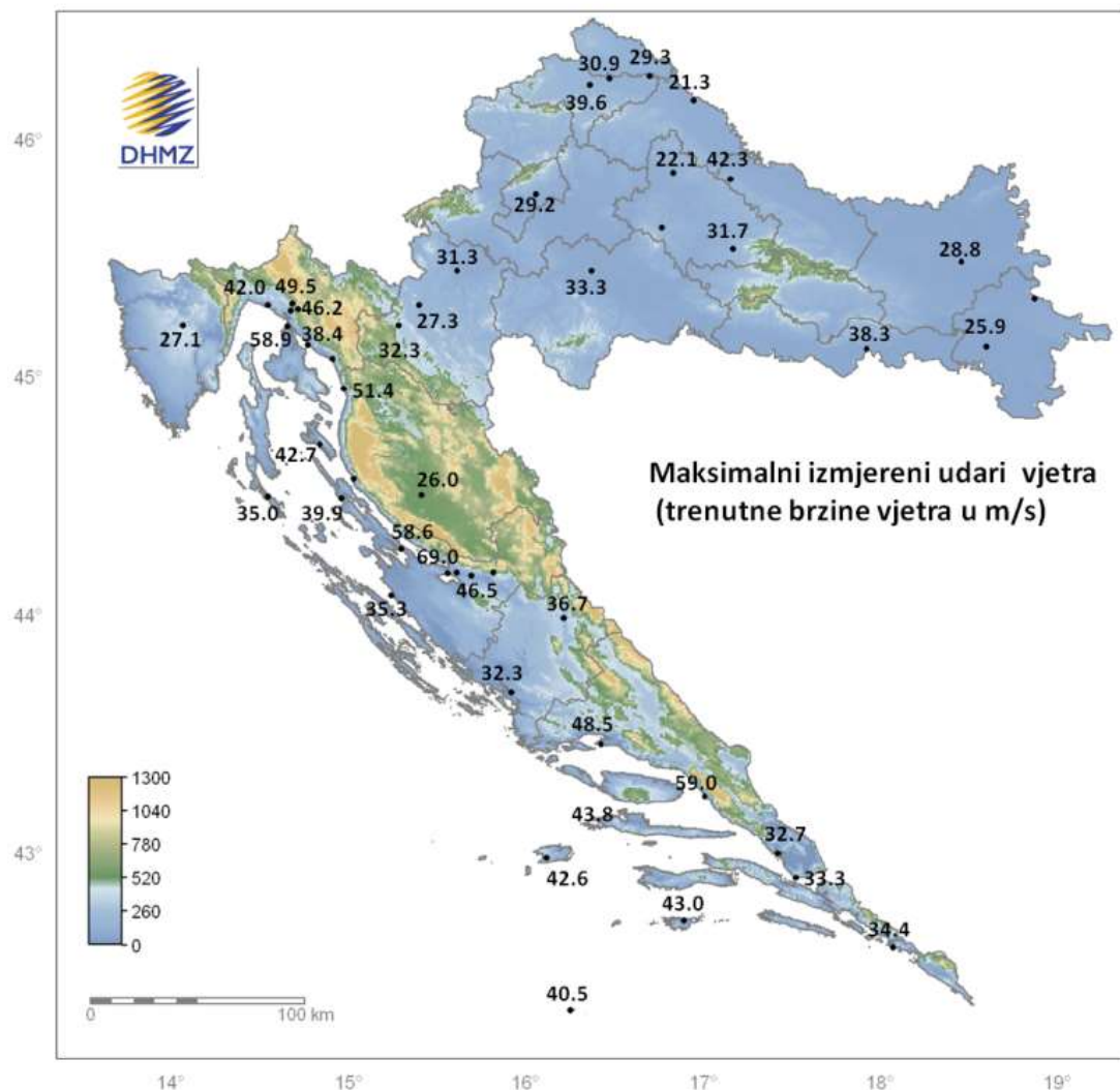
Slika 1: Maksimalni izmjereni udari vjetra (trenutne brzine vjetra) na meteorološkim postajama u Hrvatskoj Izvor podataka: Izmjene i dopune studije meteorološka podloga za potrebe procjene ugroženosti RH od prirodnih i tehničko-ehnoloških katastrofa i velikih nesreća, prosinac 2011. godine
